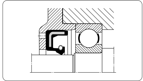
Fig 5. HMS5 seal
