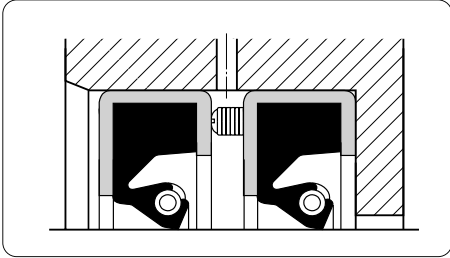
Fig 62. Spacer lugs
