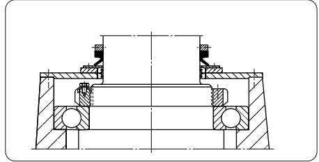
Fig 30. V-ring seal
