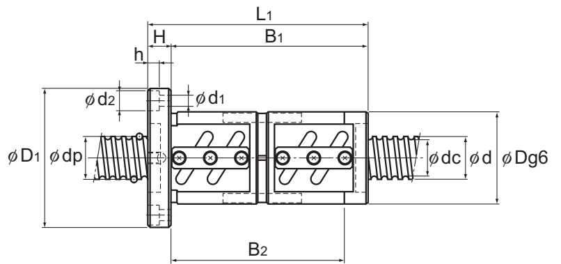
BNFN
