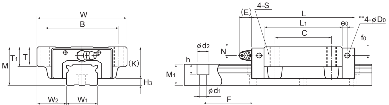
Model NRS-A
