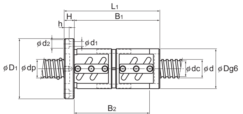
BNFN
