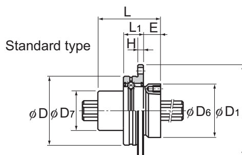
Model LTR10A
