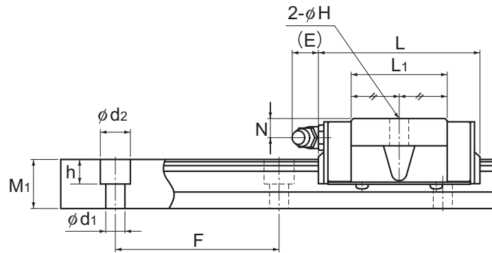
Model SR-M1SB
