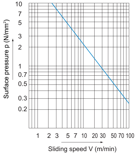
Fig.1 pV Value
