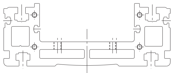
GL20
