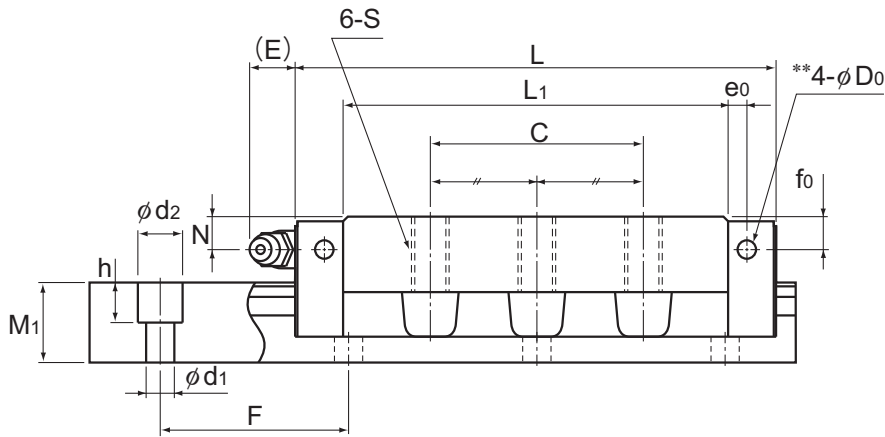
Model NR-LA
