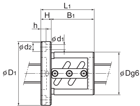
Model BNF
