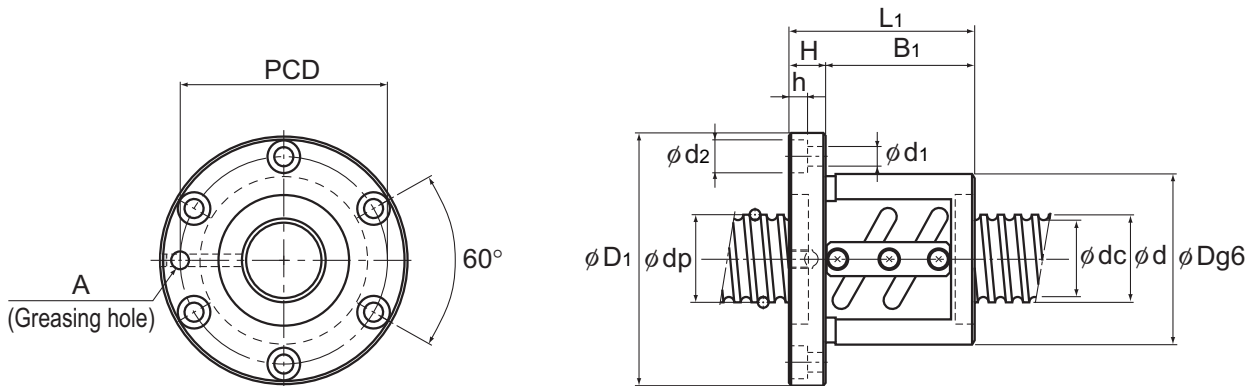
BNF
