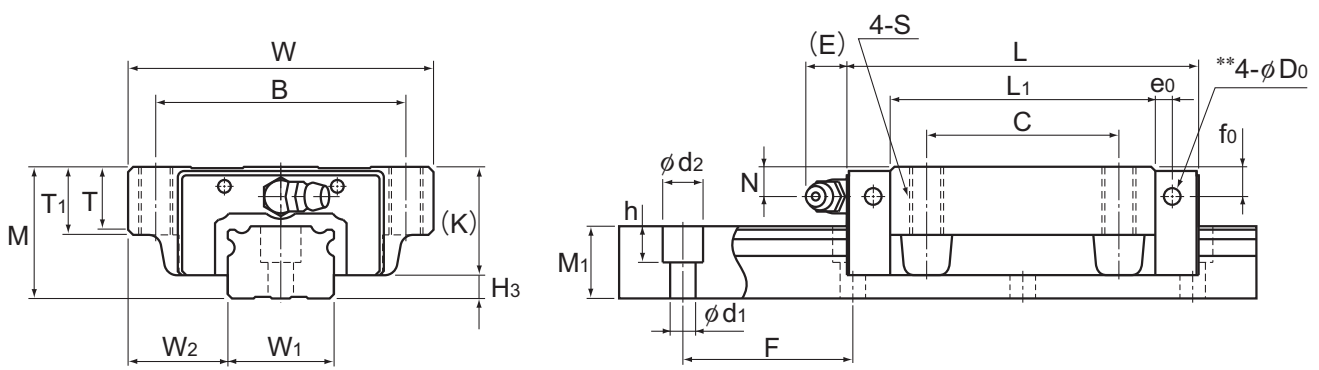
Model NR-A
