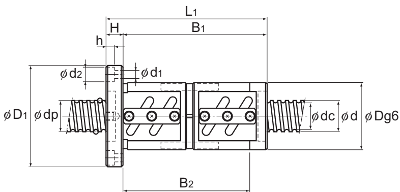
BNFN
