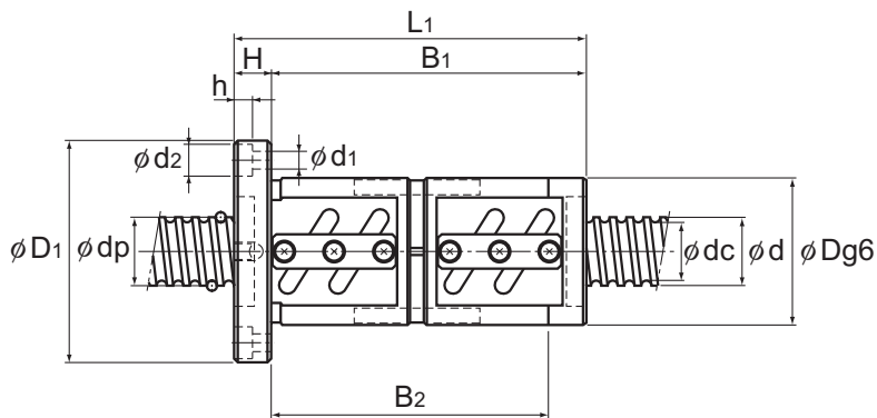
BNFN
