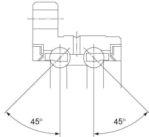
Model LTR-A
