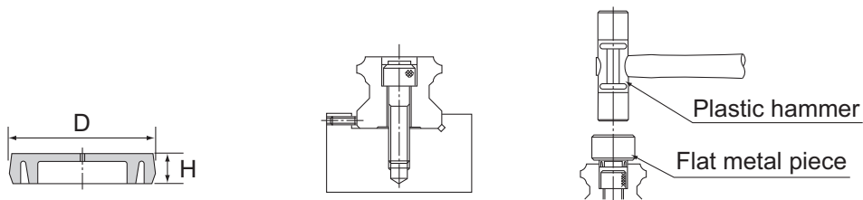
Fig.1 Cap C
