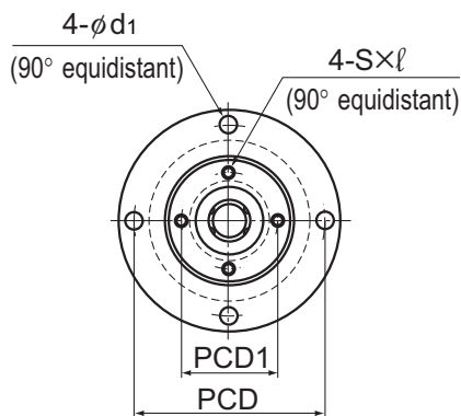
Model LTR8A Model LTR10A
