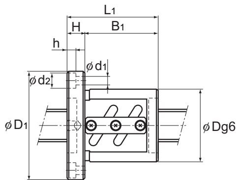
Model BNF
