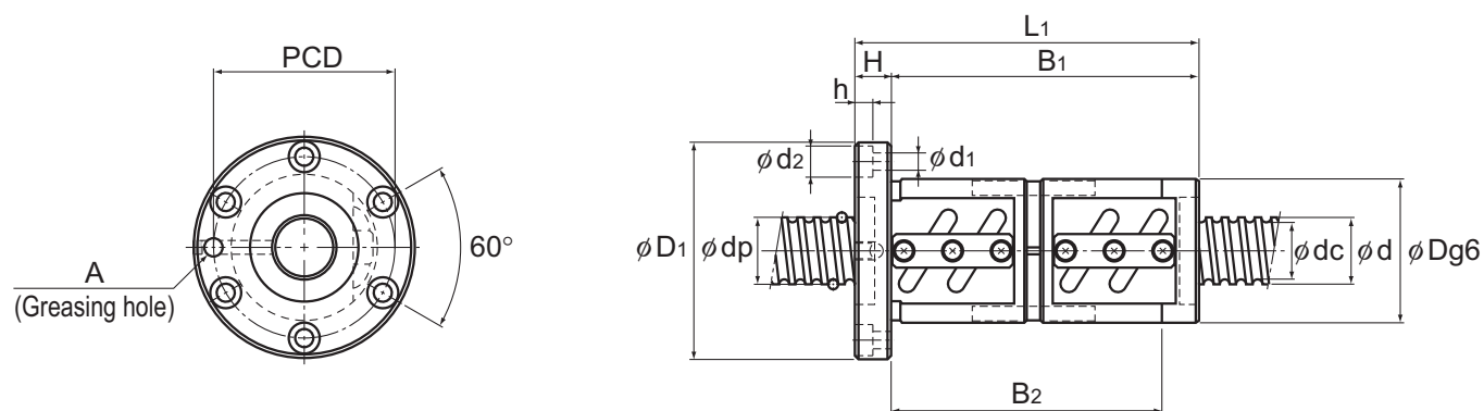
BNFN
