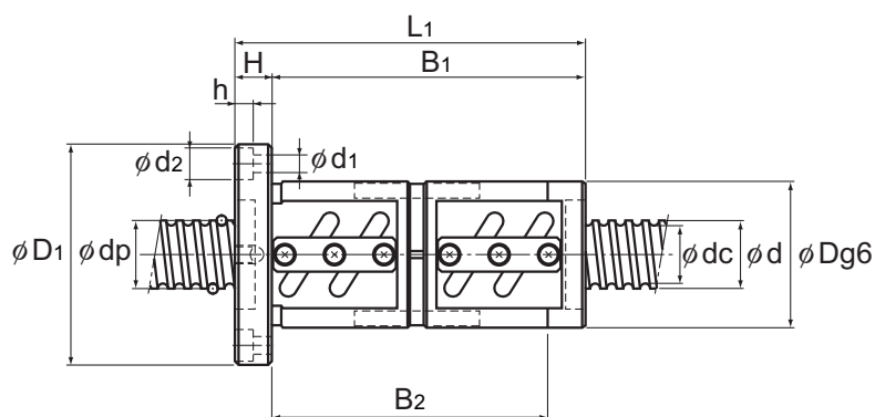
BNFN
