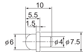
PB1021B
