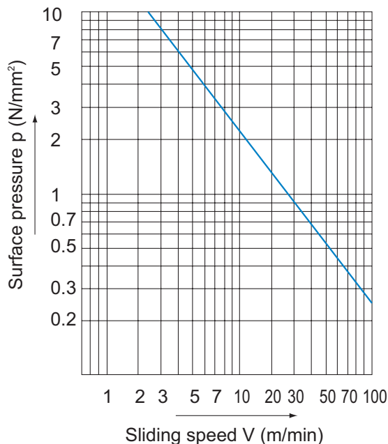
Fig.1 pV Value
