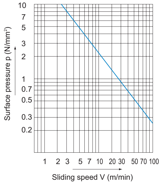
Fig.1 pV Value
