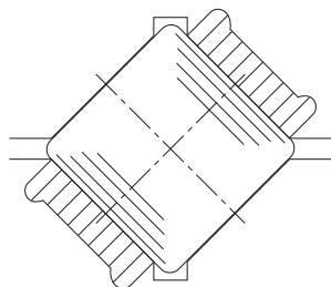
Нагружаемые области симметричны С фиксирующим сепаратором
