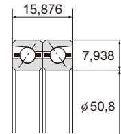
Радиально-упорный подшипник
