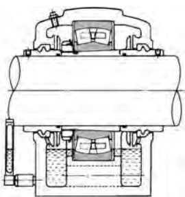
Смазка погружением: не для высоких скоростей
