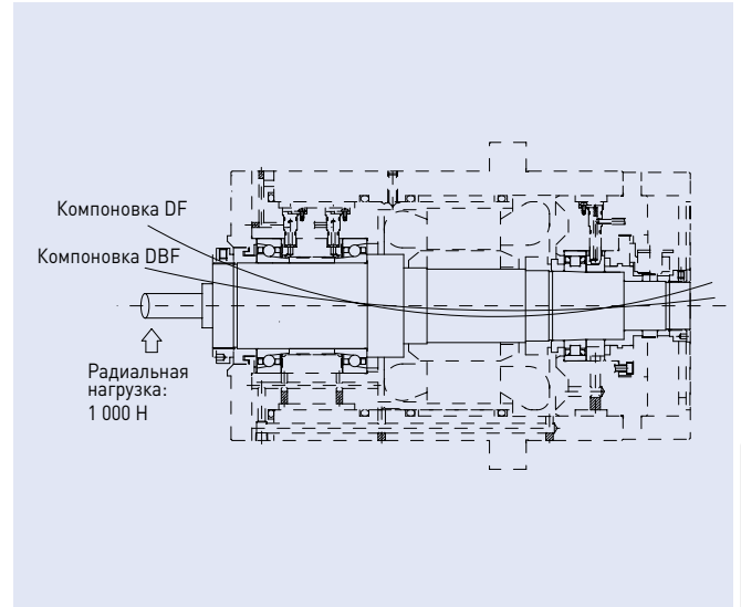
Рис. 3.6 Комбинации радиально-упорных шариковых подшипников
