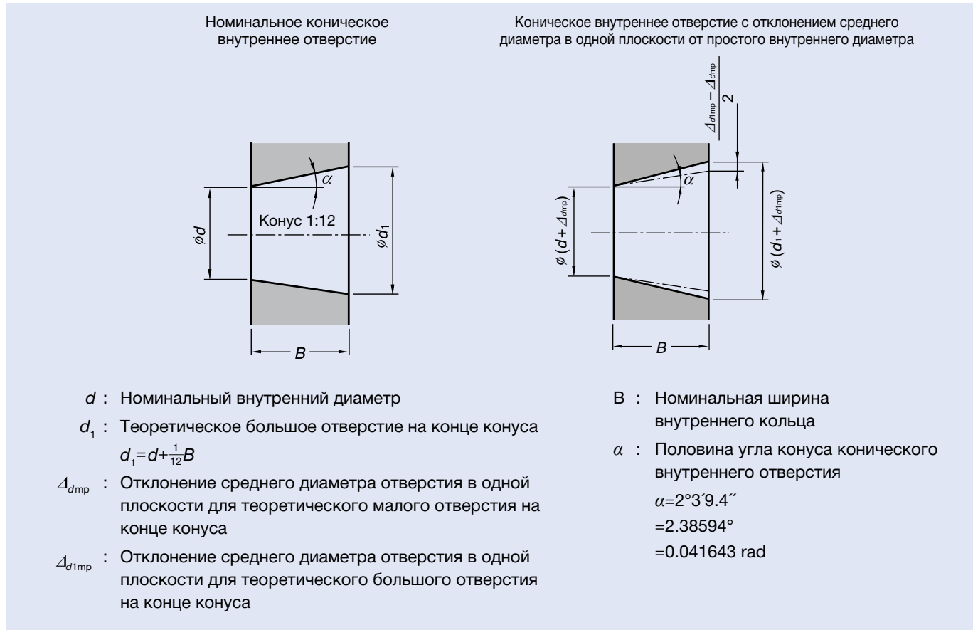
Рис. 7.3 Допустимые отклонения конического внутреннего отверстия
