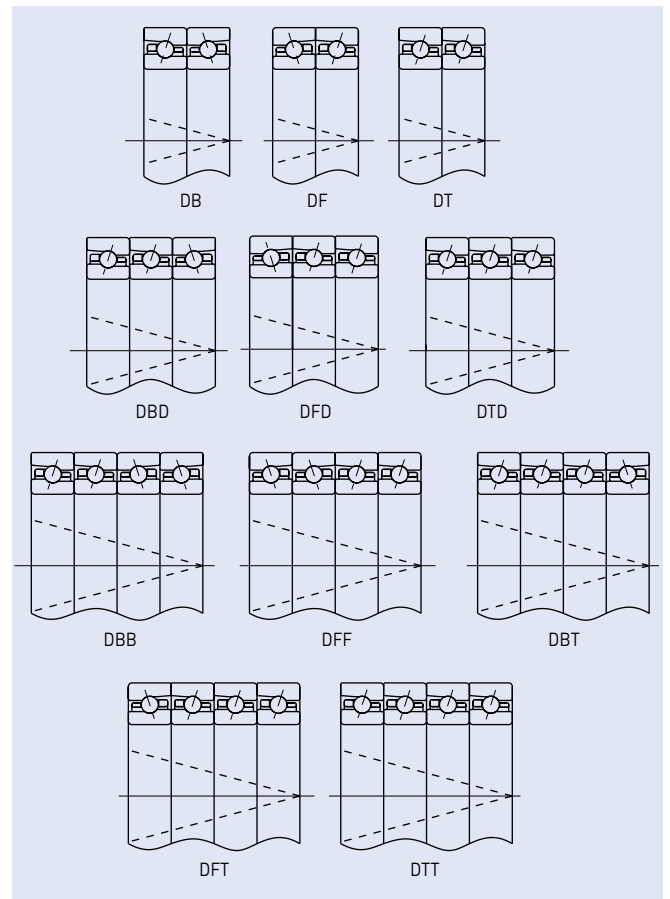
Рис. 3.6 Комбинации радиально-упорных шариковых подшипников
