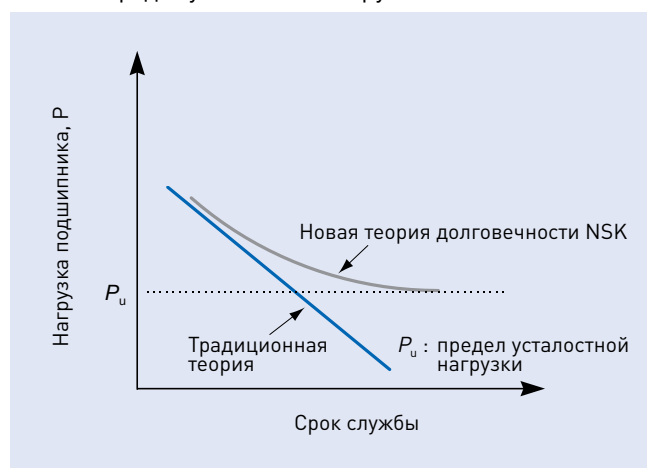
Рис. 1.2 Новая теория долговечности NSK, учитывающая предел усталостной нагрузки
