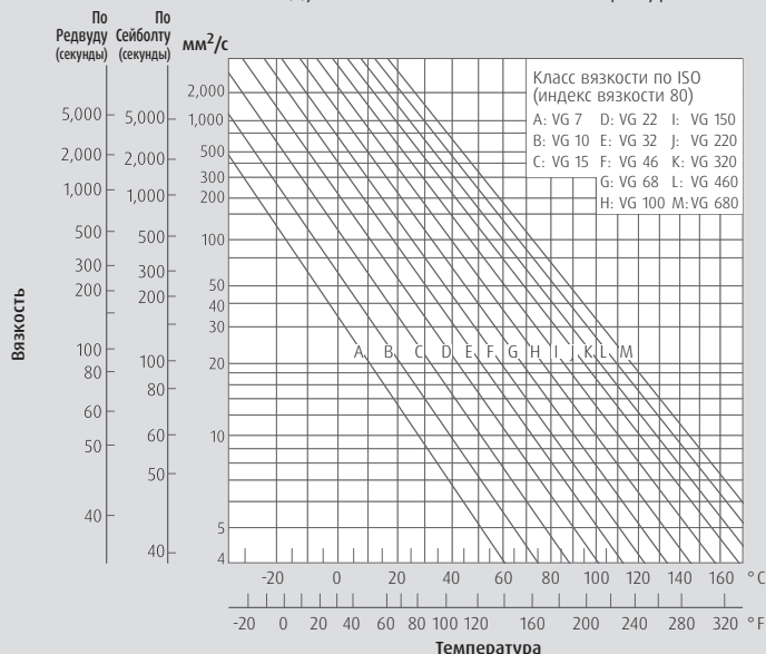
Рис. 1 Зависимость между вязкостью масла и температурой
