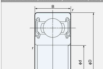
Бесконтактное резиновое уплотнение (NKE9)
