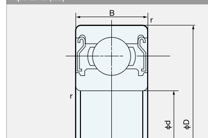
Крышка (ZE)
