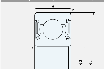
Контактное резиновое уплотнение (NSE9)
