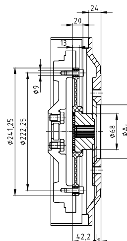
Yanmar TMV-Series
