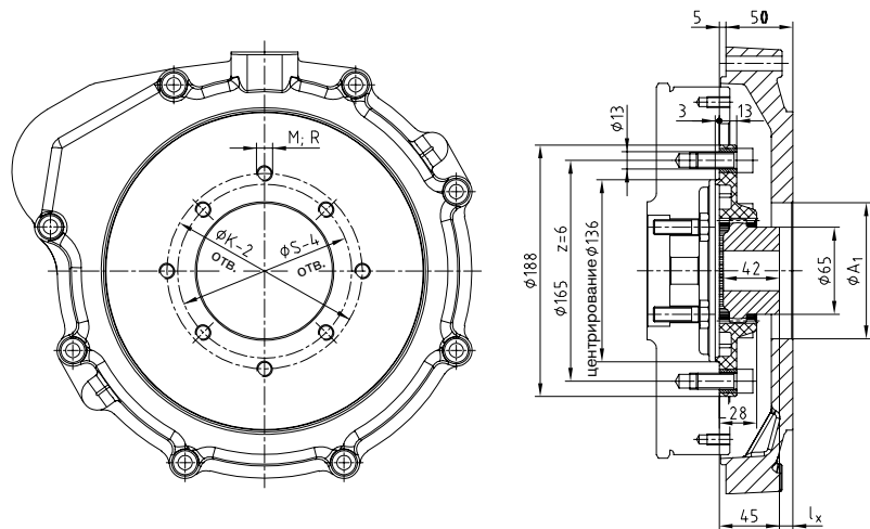
BoWex® 48 FLE-PA Ø 188 / корпус насоса
