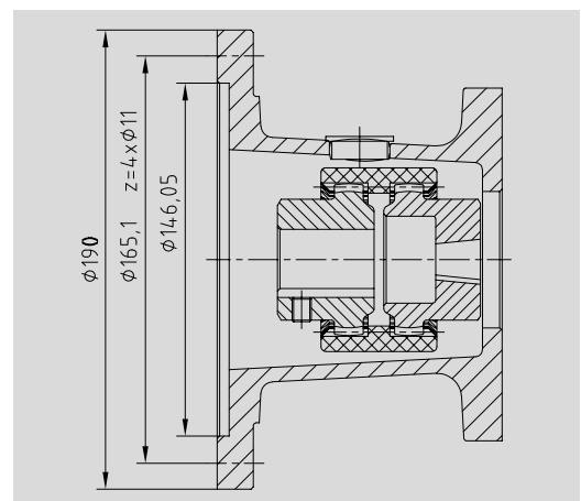
BoWex® Соединительная муфта Тип M28 и M32 Соединение в соотв. с SAE J609A
