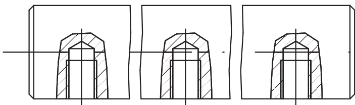
Foratura radiale Radial drilling
