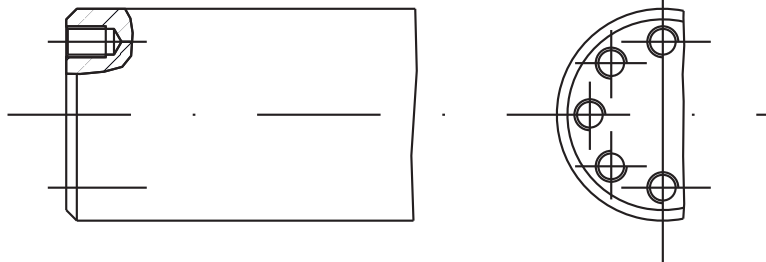
Foratura assiale circolare Circular axial drilling
