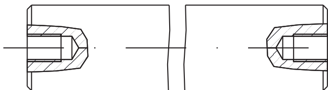
Foratura assiale Axial drilling
